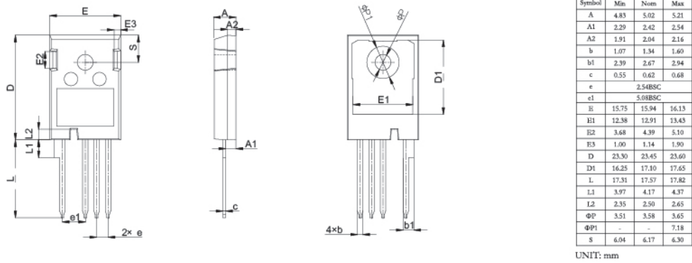
TO-247-4L
