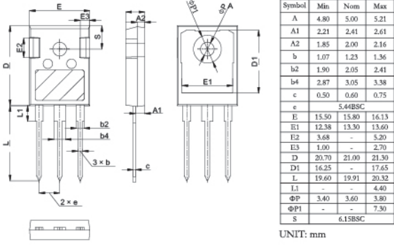
TO-247-3L
